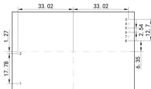
封装图
