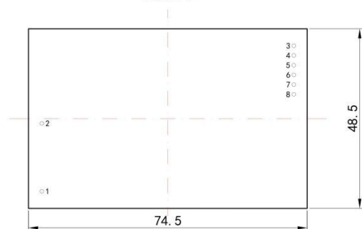
俯视图
