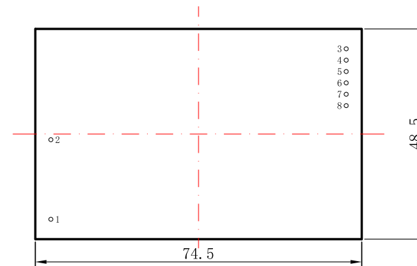
俯视图
