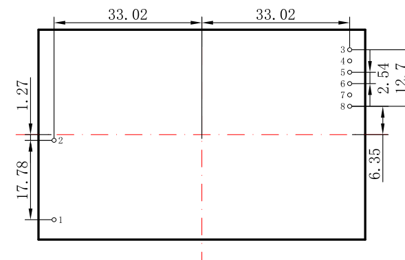
封装图
