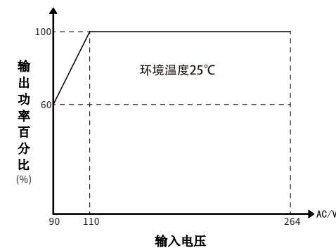
输入电压降额曲线图
